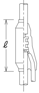
分岐処理詳細図 (例:1分岐処理)
