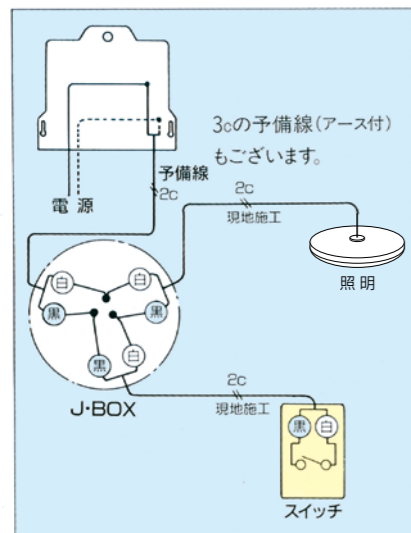
予備線を利用して照明回路を追加する場合
