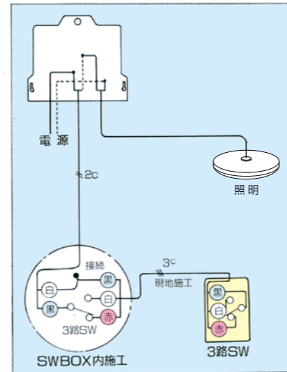
片切回路を3路回路に変更する場合
