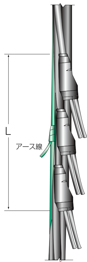
アース付2分岐 分岐処理図(例) (CVT)
