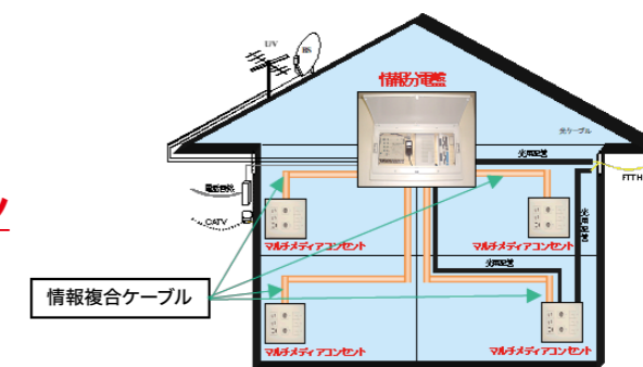
情報複合ケーブルを用いた配線方法
